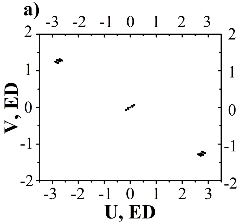
Рисунок 2.1 — Реализованные покрытия uv -плоскости в наблюдениях от 11.01.2014 мазера \text{H}_2\text{O} в области звёздообразования NGC 2071 IRS 1 за весь сеанс наблюдений от 17:00 час до 18:00 час UTC: а) наземно-космические базы; б) наземные базы в увеличенном масштабе. Телескопы: 10-м Ра (SRT), 32-м Мс, 32-м Тр, 64-м К1 (рис.1 из работы Щуров и др. 2021 [87]).
