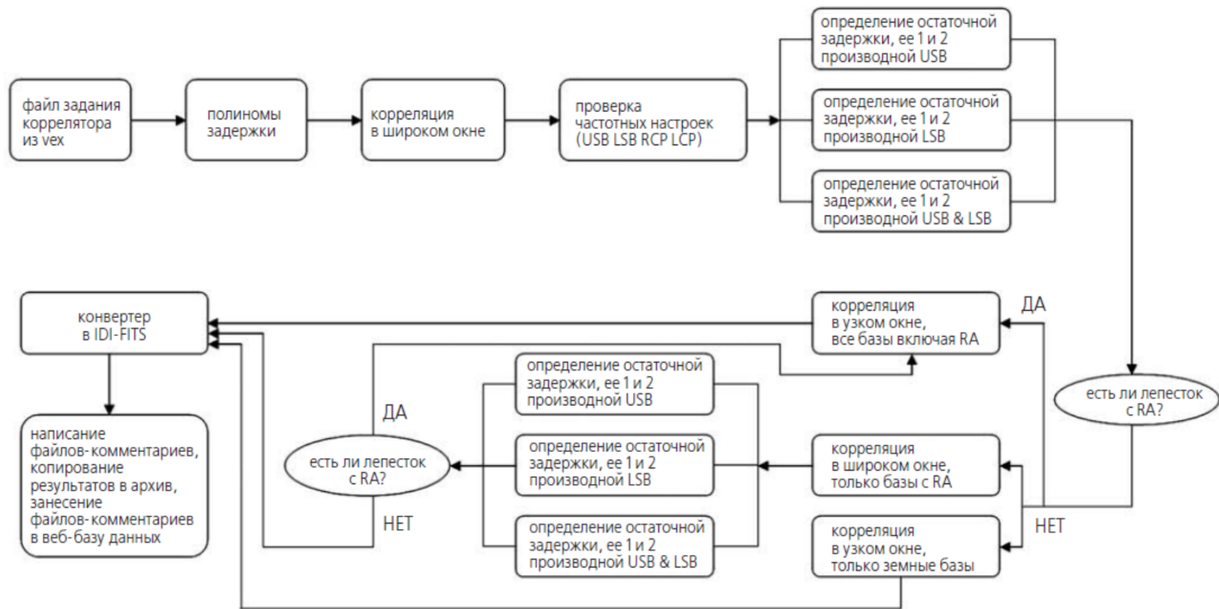
Рисунок 3.1 — Порядок обработки данных на корреляторе АКЦ, полученных в результате измерений, проведённых на наземно-космическом интерферометре в рамках проекта “РадиоАстрон” (иллюстрация из диссертационной работы Андрианова [88]).
