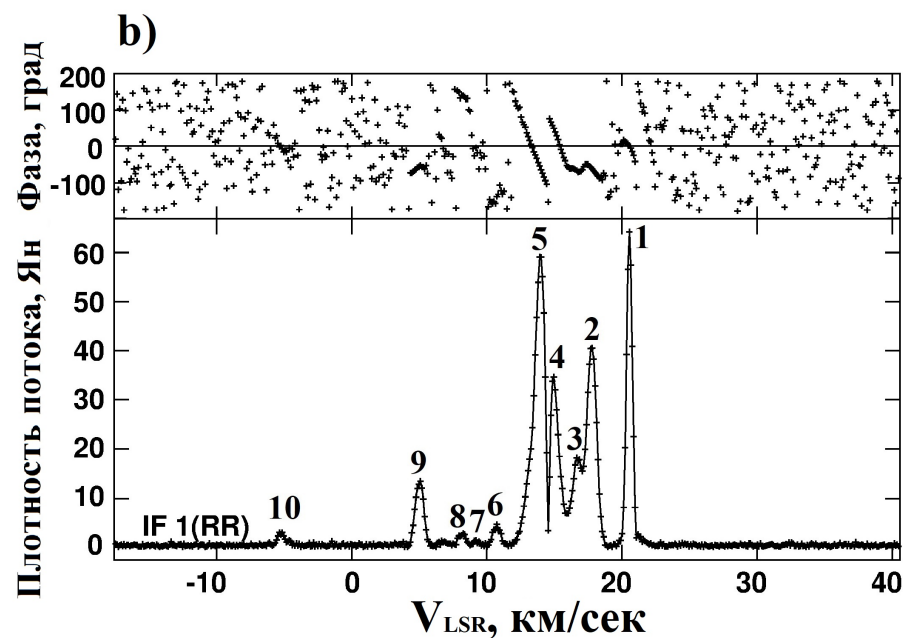
Рисунок 2.6 — а) кросс-корреляционный спектр мазера \text{H}_2\text{O} в источнике NGC 2071 IRS 1 в каналах ПОСЛЕ применения фазовой калибровки по калибровочному каналу (деталь №1). б) кросс-корреляционный спектр мазера \text{H}_2\text{O} в источнике NGC 2071 IRS 1 в скоростях ПОСЛЕ применения фазовой калибровки по калибровочному каналу (деталь №1, рис.6 из работы Щуров и др. 2021 [87])).
