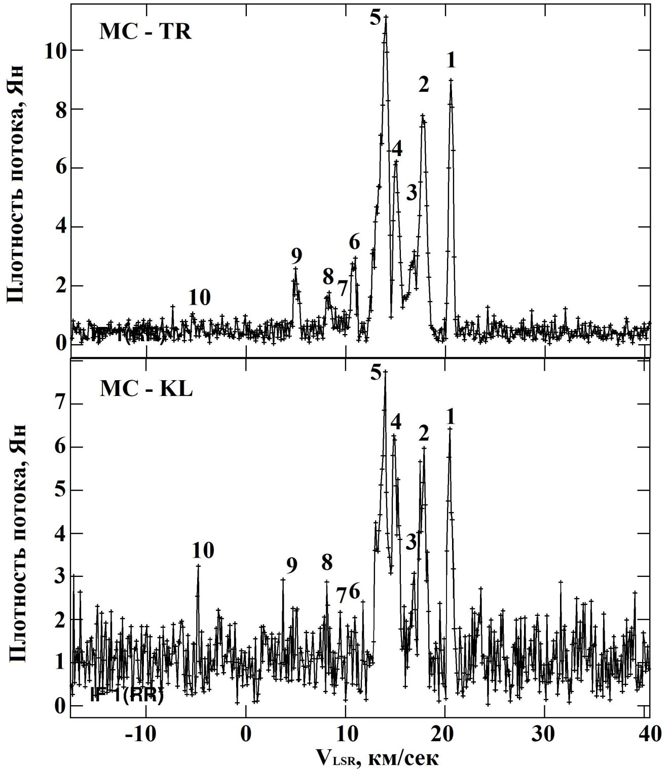
Рисунок 2.11 — Кросс-корреляционный спектр источника NGC 2071 IRS 1 (в скоростях): верхний - на короткой базе интерферометра Мс-Тр; нижний - на длинной базе интерферометра Мс-Кл. Нумерация спектральных деталей приведена в соответствии с кросс-корреляционным спектром в каналах – см. рис. 2.6 (рис.10 из работы Щуров и др. 2021 [87]).
