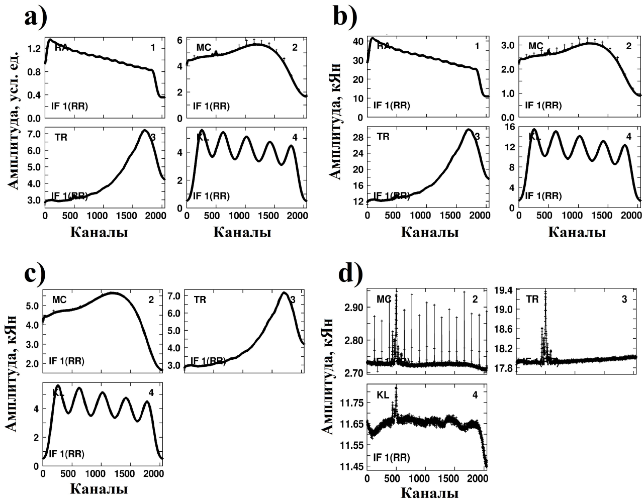
Рисунок 2.2 — а) Первичные некалиброванные автокорреляционные спектры мазера \text{H}_2\text{O} в источнике NGC 2071 IRS 1 в полной полосе регистрации 16 МГц; б) те же спектры после применения данных из штатных калибровочных таблиц; в) вид полосы пропускания при наблюдениях калибровочного квазара на антеннах наземной сети; д) автокорреляционные спектры мазера при наблюдениях на наземных телескопах с применением корректировки полосы пропускания по квазару. Представлены наблюдения только на 3-х наземных антеннах - в наблюдениях квазара SRT не участвовал (см. текст). Рис.2 из работы Щуров и др. 2021 [87].
