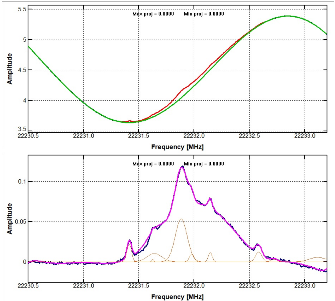
Рисунок 3.4 — Автоспектр источника NGC 2071 IRS 1 на станции «Калязин» (РТ-64). Сверху - до коррекции полосы полиномом, снизу - после коррекции.
