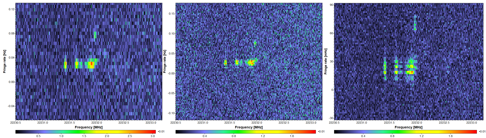
Рисунок 3.8 — Диаграмма “Частота интерференции - частота” для источника NGC 2071 IRS 1 в сеансе rax07ar от 11.01.2014 для трёх разных периодов времени на базе “Медицина - Калязин”. Слева - диаграмма для 3-ёх минут, посередине - для 5-ти минут, справа - для 10-ти минут (иллюстрация обработки данных для гл.2).
