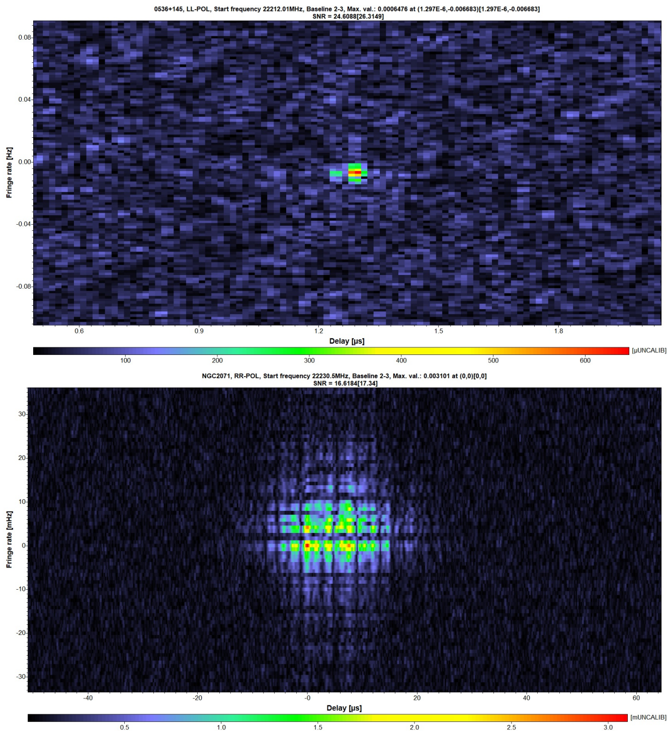
Рисунок 3.2 — Сверху - корреляционный отклик квазара TXS 0536+145. Корреляция во всей полосе частот даёт узкий корреляционный отклик - можно определить координаты максимума отклика, что даёт возможность скомпенсировать геометрические задержки для телескопов. Снизу - корреляционный отклик мазера в области NGC 2071 IRS 1. Корреляция в нескольких узких интервалах частот даёт множество широких корреляционных откликов, сложно определить координаты какого-либо максимума, пик «размыт» по обеим осям (иллюстрация обработки данных для гл.2).
