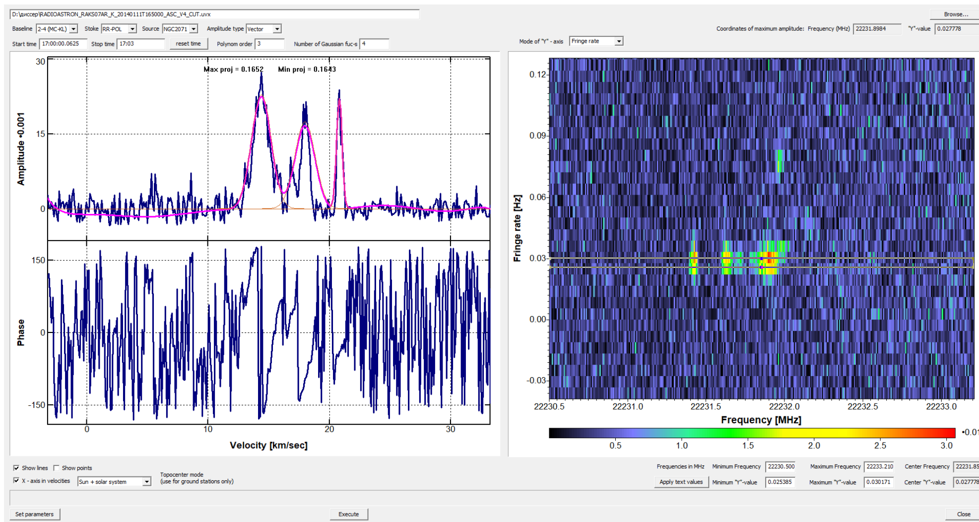
Рисунок 3.7 — Главное окно программы LineViewer, справа - Вид корреляционного отклика системы на диаграмме “Fringe rate - frequency” для наблюдений источника NGC 2071 IRS 1 для сеанса raks07ar от 11.01.2014 г. на базе “Медицина - Калязин”, время усреднения - 3 минуты (иллюстрация обработки данных для гл.2). Слева - амплитуда (сверху) и фаза (снизу) кросс-корреляционного спектра на выделенной частоте интерференции, по оси абсцисс - лучевая скорость относительно наблюдателя (км/с).
