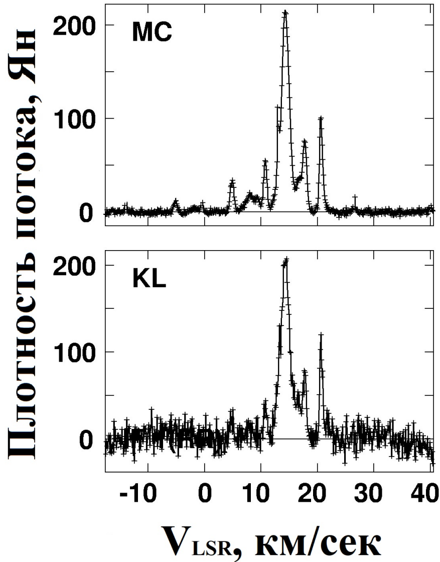
Рисунок 2.3 — Автокорреляционные спектры мазера \text{H}_2\text{O} в источнике NGC 2071 IRS 1 с полной амплитудной калибровкой; по оси X – скорости спектральных деталей, по оси Y - калиброванный поток в Ян (рис.3 из работы Щуров и др. 2021 [87]).
