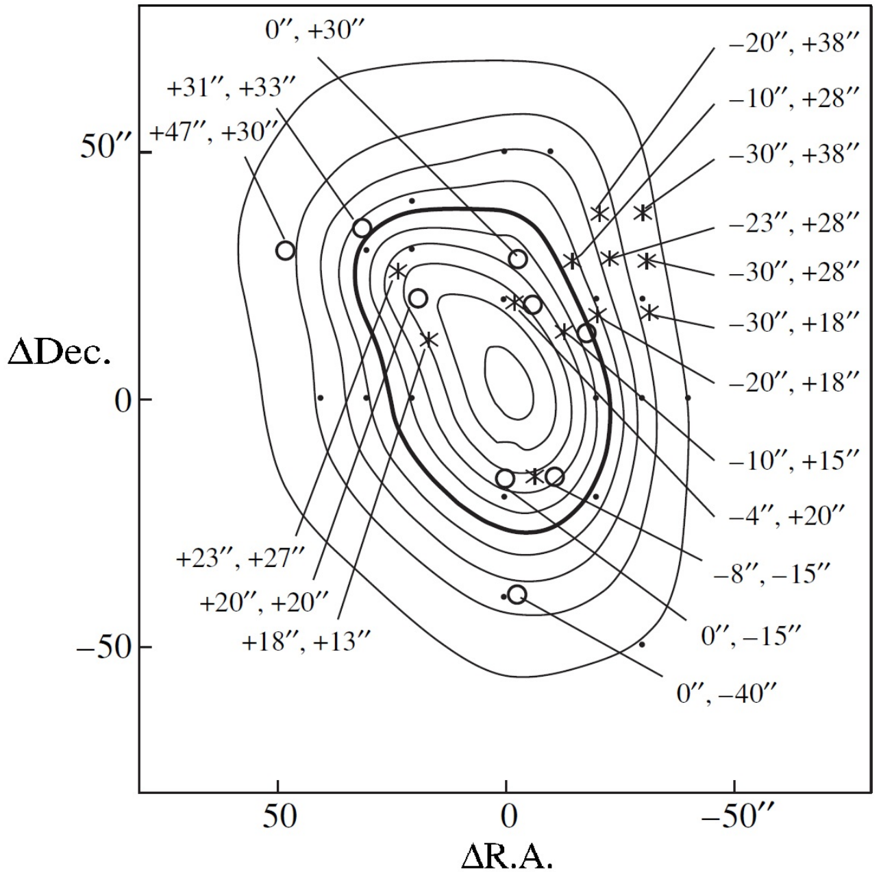
Рисунок 1.1 — Карта L379 IRS1. Кругами обозначены направления, наблюдавшиеся в 2003 г, звездочками — в 2007 г. Контуры показывают распределение интегральной интенсивности в линии CS J = 2 - 1 (рис.1 из работы Щуров & Каленский 2016 [50]).
