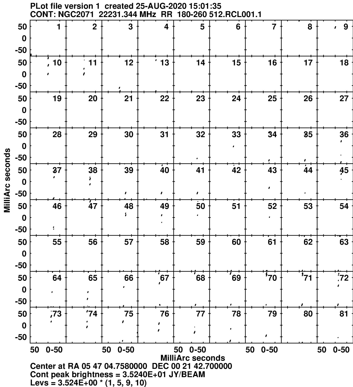
Рисунок 2.7 — Развёрнутая карта для части спектра, в которой присутствуют мазерные линии - каналы №№180-260: для каждого канала в двумерном изображении с координатами по прямому восхождению по оси X и по склонению по оси Y. Размер карты для каждого канала 512×512 пикселей (иллюстрация, в работе Щуров и др. 2021 [87] присутствует ссылка на изображение на сайте АКЦ).
