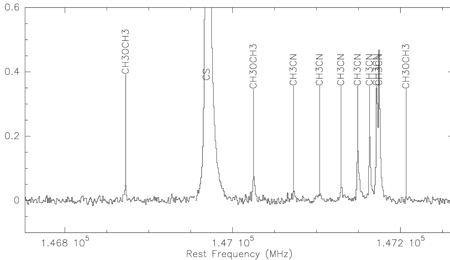
Рисунок 1.2 — Спектр L379 IRS1 в направлении -8'' , -15'' (рис.2 из работы Щуров & Каленский 2016 [50]).
