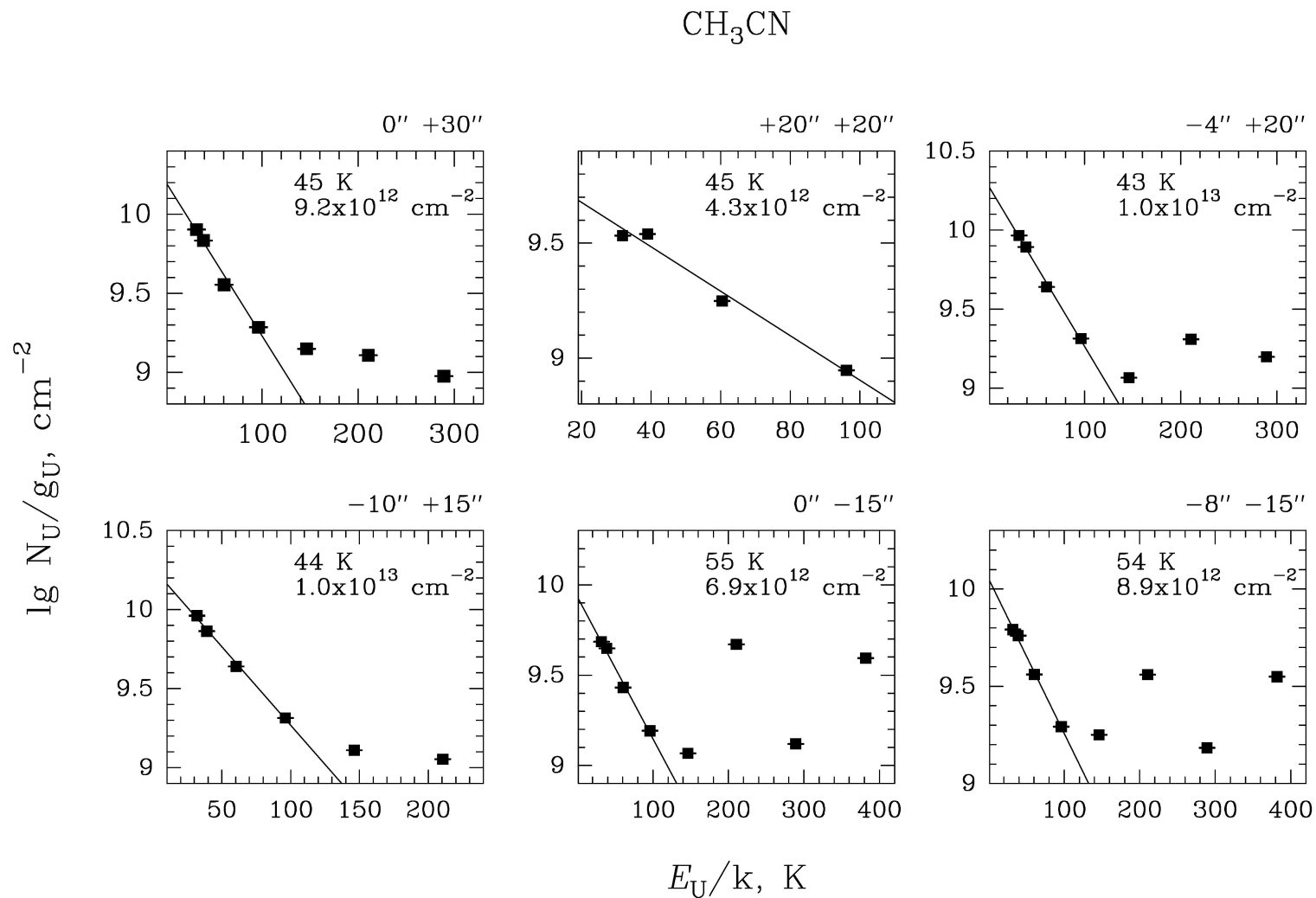
Рисунок 1.5 — Вращательные диаграммы, построенные по линиям метилцианида 8_K - 7_K на частоте 147 ГГц. Для линий K = 4 - 7 не выполняются условия, при которых вращательные диаграммы применимы (см. раздел 1.5) (рис.5 из работы Щуров & Каленский 2016 [50]).
