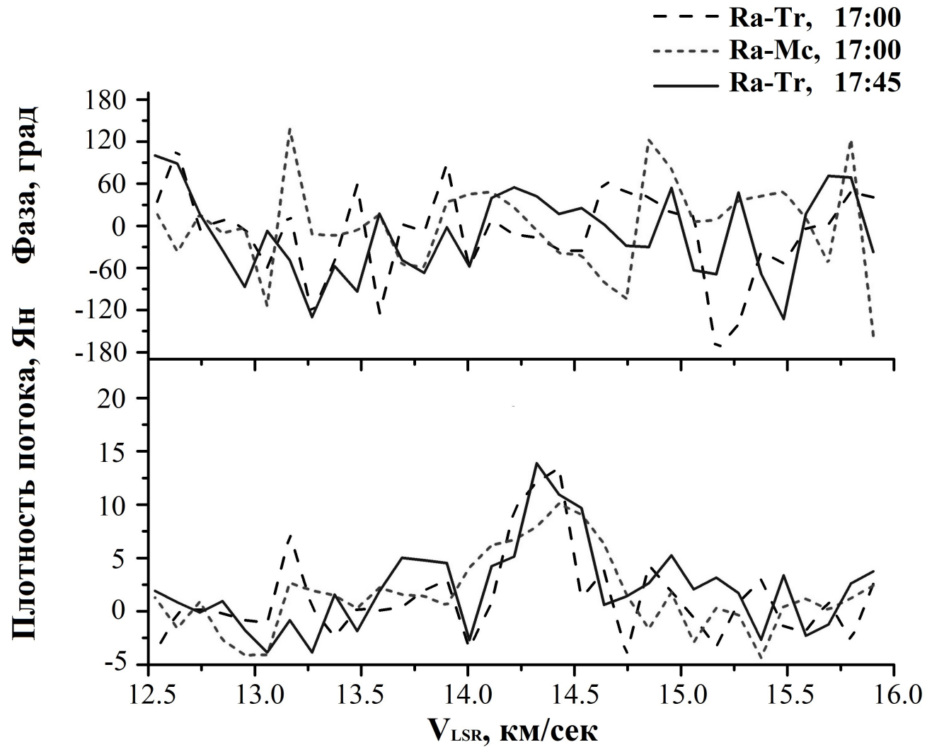
Рисунок 2.9 — Амплитуда (нижняя панель) и фаза (верхняя панель) корреляции на базе SRT-Mc (один 15-минутный скан) и на базе SRT-Tr (два 15-минутных скана), соответствующая спектральной детали №5_1 на скорости 14.3 км/с. Представлены данные в правой поляризации (рис.8 из работы Щуров и др. 2021 [87]).
