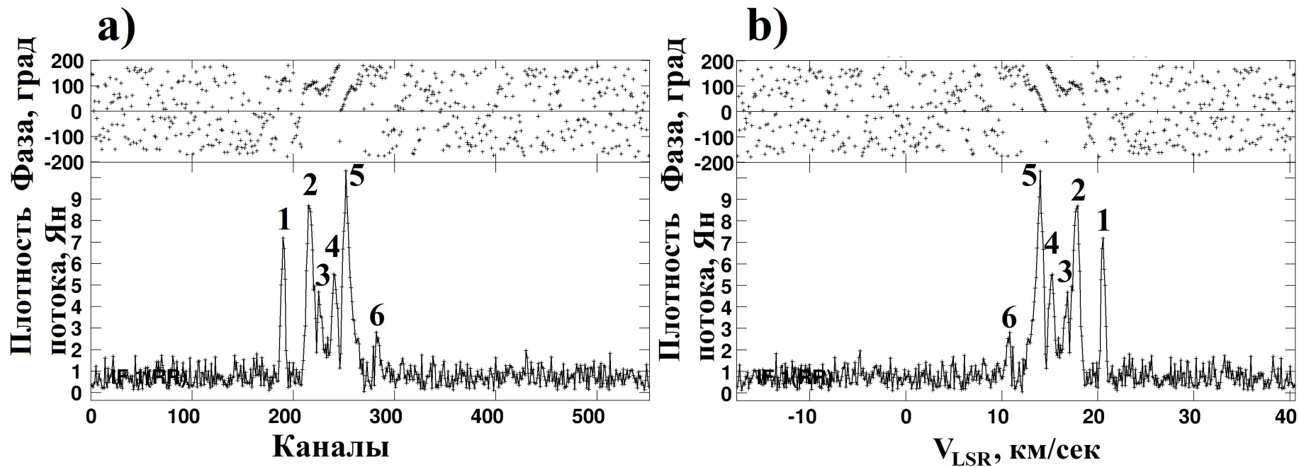
Рисунок 2.4 — а) Кросс-корреляционный спектр мазера H_2O в NGC 2071 IRS 1 на наземной сети в каналах с полной амплитудной калибровкой ДО исправления фазы по калибровочному каналу (соответствующая спектральная деталь отмечена как №1); б) тот же спектр в скоростях (рис.4 из работы Щуров и др. 2021 [87]).
