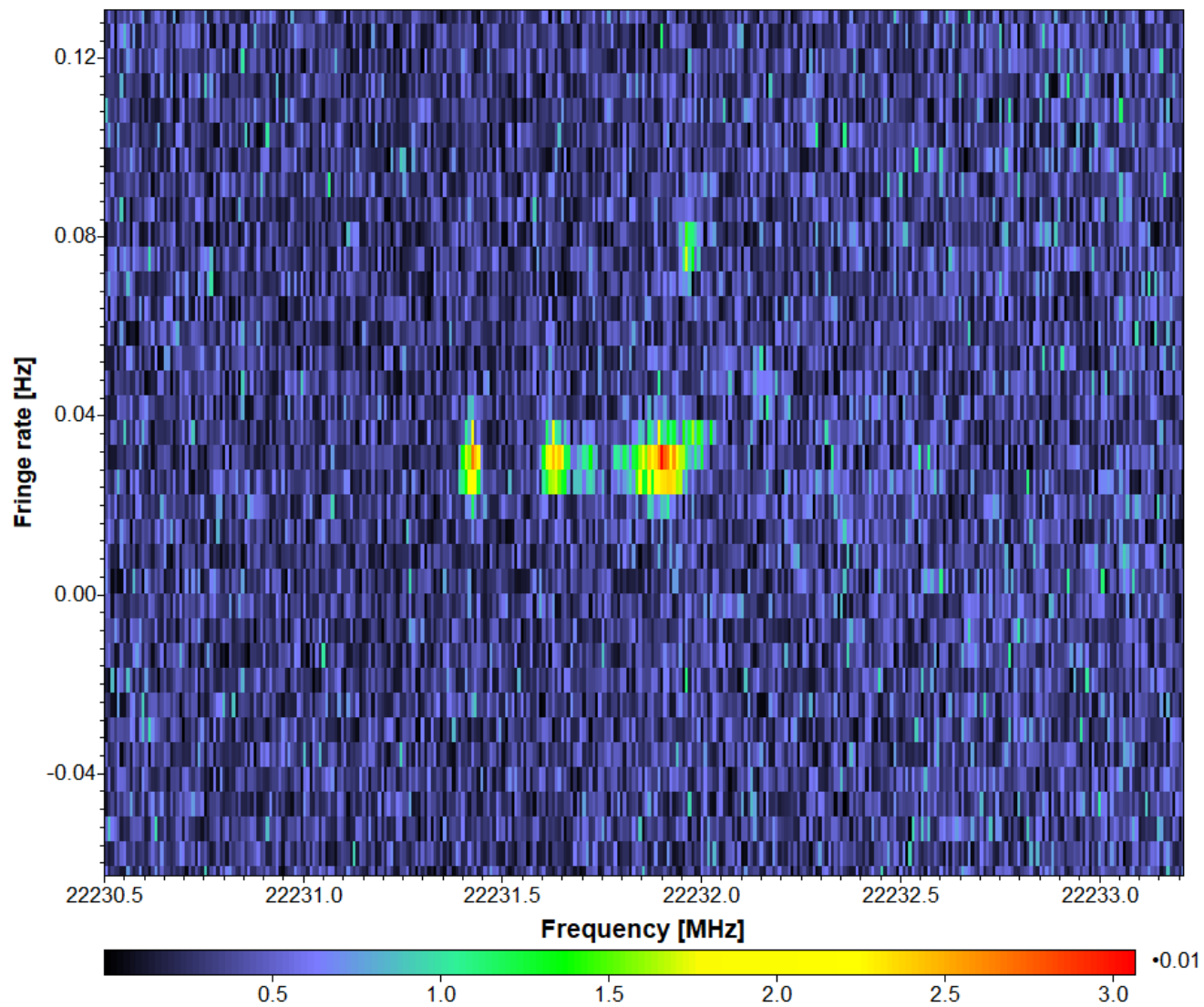
Рисунок 3.5 — Вид корреляционного отклика системы на диаграмме “Fringe rate - frequency” для наблюдений источника NGC 2071 IRS 1 для сеанса raks07ar от 11.01.2014 г. на базе “Медицина - Калязин”, время усреднения - 3 минуты (иллюстрация обработки данных для гл.2).
