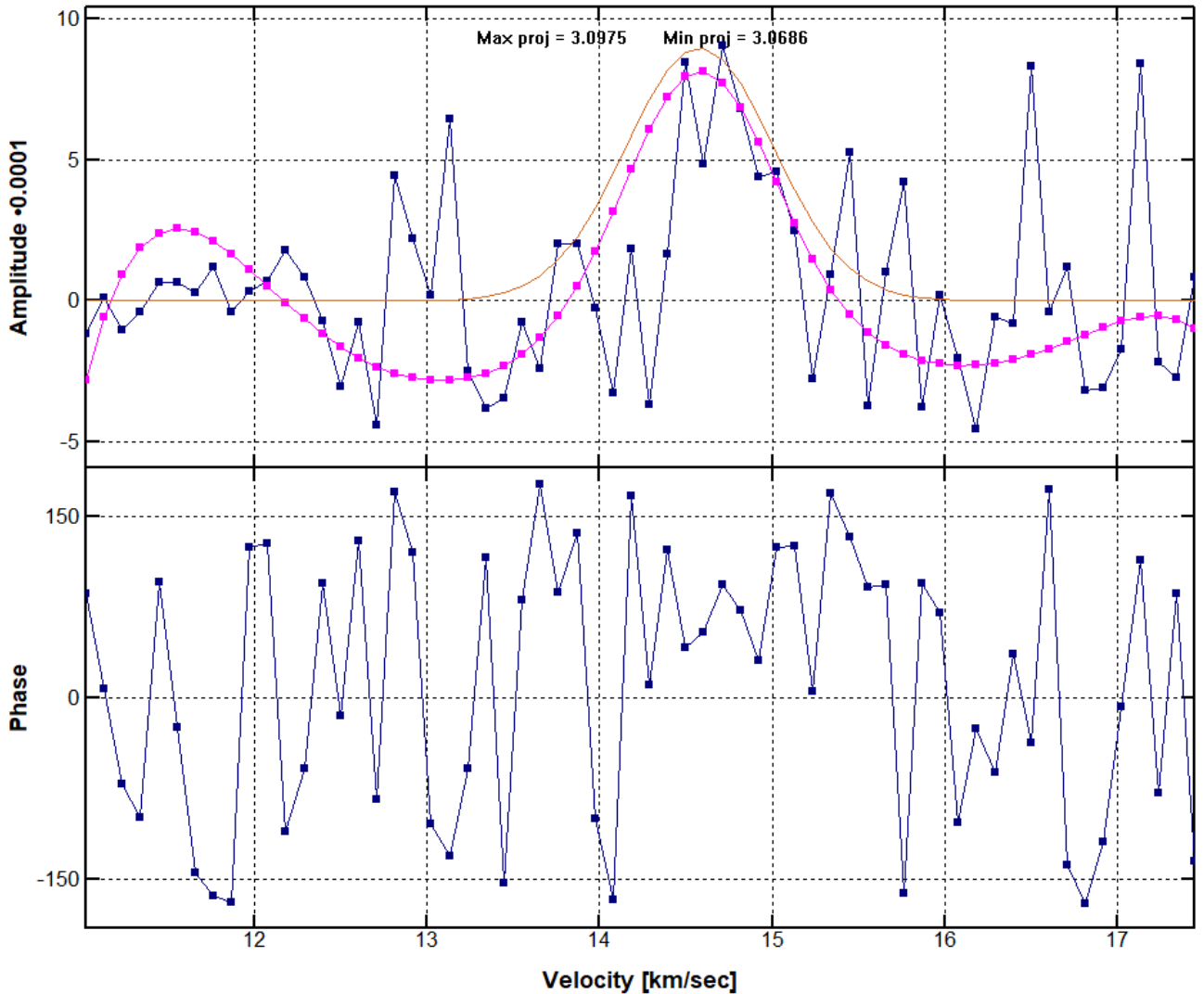
Рисунок 3.6 — Корреляционный отклик источника NGC 2071 IRS 1 в сеансе raks07ar от 11.01.2014 г. на базе “РадиоАстрон - Медицина” и его аппроксимация функцией Гаусса. Сверху - амплитуда, снизу - фаза корреляционного отклика. По оси абсцисс представлены лучевые скорости, по оси ординат для верхнего поля - условные единицы амплитуды, для нижнего - градусы (иллюстрация обработки данных для гл.2).
