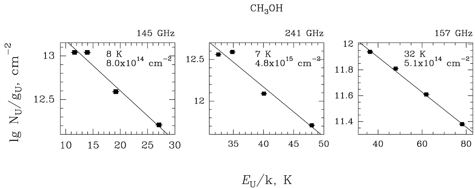
Рисунок 1.3 — Вращательные диаграммы, построенные по линиям метанола в направлении -4'' , +20'' (рис.3 из работы Щуров & Каленский 2016 [50]).
