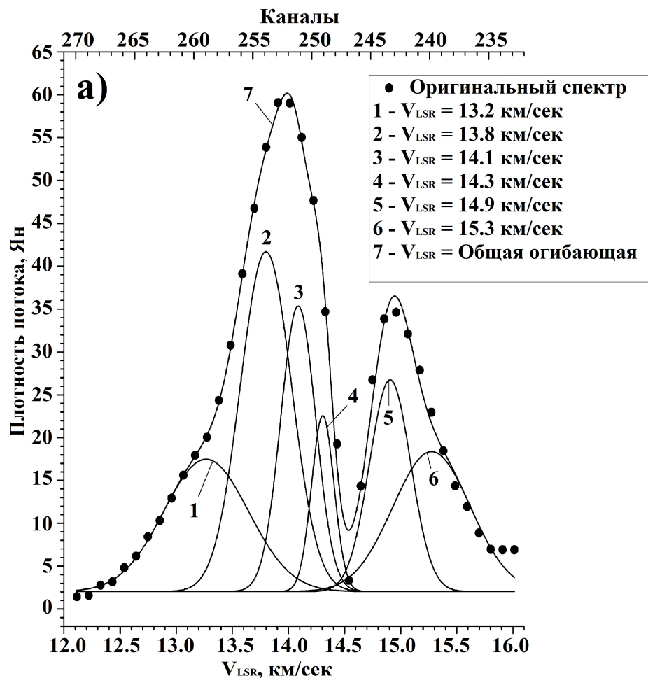
Рисунок 2.10 — а) аппроксимация суммой Гауссиан участка спектра для скоростей 12.0 – 16.0 км/с (каналы №233-270, спектральные детали №4-5, выполнено в программе ORIGIN; б) комбинированная карта для компонентов с максимумами на скоростях 13.8, 14.1 и 14.3 км/с - спектральная деталь №5. Размер карты (512 × 512) пикселей (рис.9 из работы Щуров и др. 2021 [87]).
