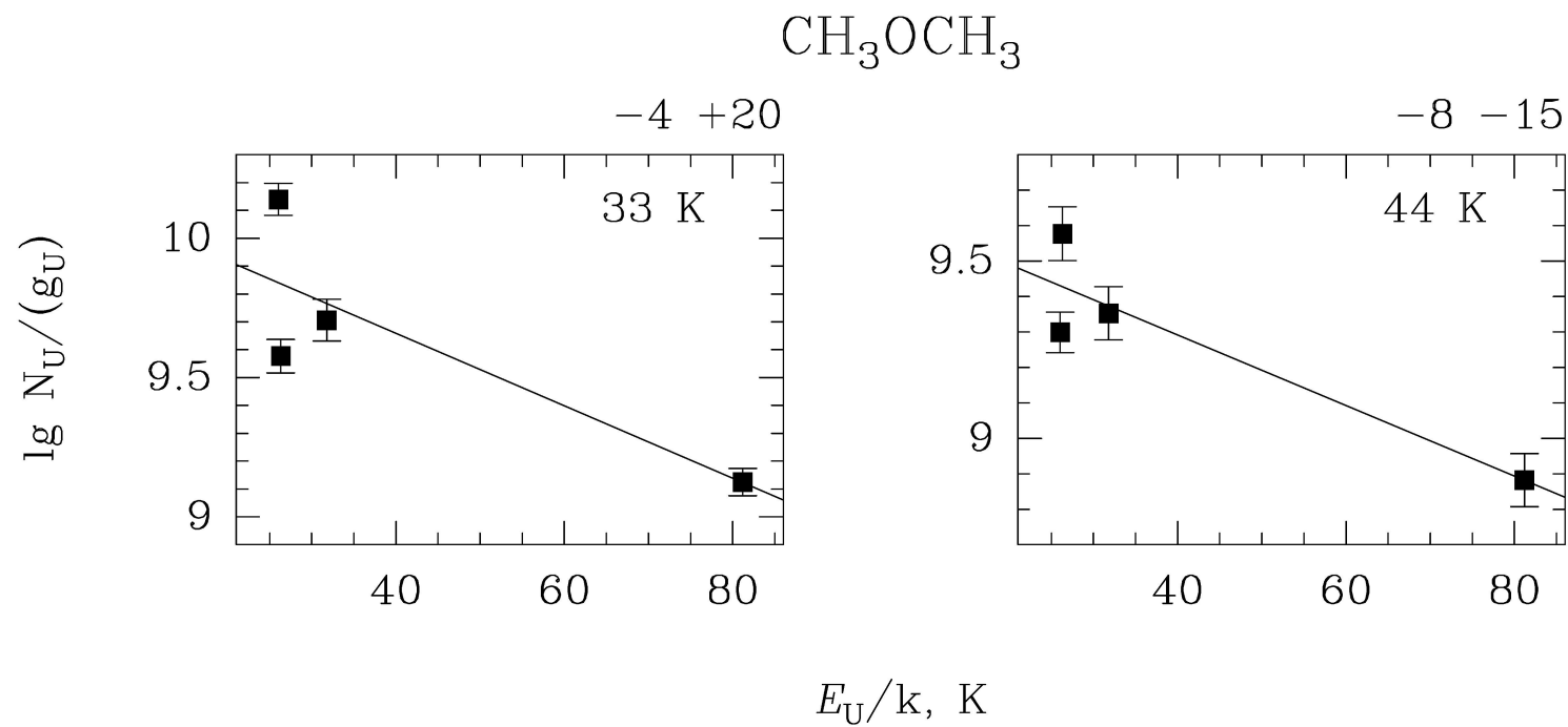
Рисунок 1.6 — Вращательные диаграммы, построенные по линиям диметилэфира (рис.6 из работы Щуров & Каленский 2016 [50]).
